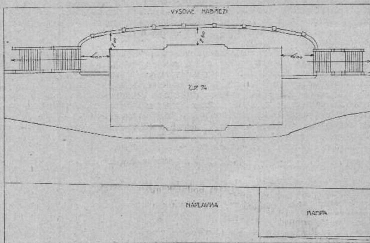
Návrh technického úřadu města Smíchova na úpravu okolí zahradního domku č. p. 74 v býv. botanické zahradě na Smíchově.
